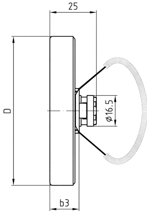
Anschluss axial, mit Befestigungsfedern
