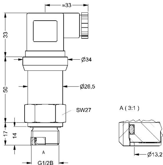
DMU 03 VM - Anschluss G1/2B DIN 3852-Form E mit vorgezogener Membrane
