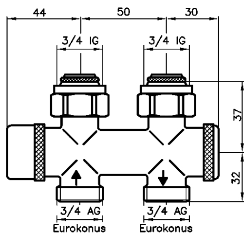
456-DP, Durchgang – Ausführung G \frac{3}{4} -Innengewinde
