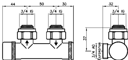
456-DP, Eck – Ausführung G \frac{3}{4} -Innengewinde
