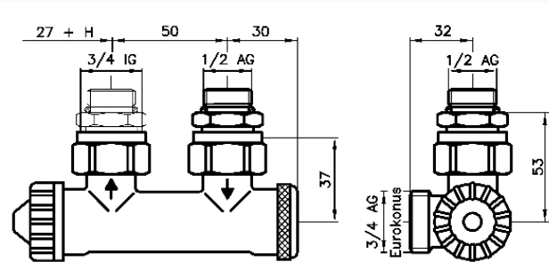
Vario DP, Eck – Ausführung G \frac{1}{2} Aussengewinde
