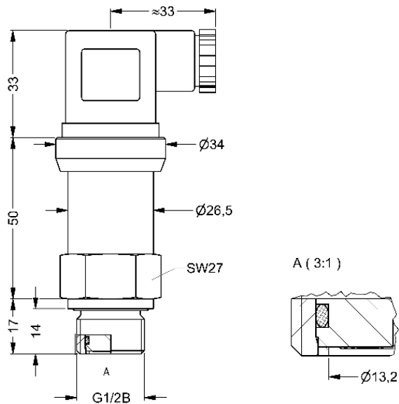
DMU 03 VM - Anschluss G1½B DIN 3852-Form E mit vorgezogener Membrane
