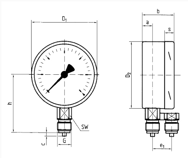
Masse (mm)
