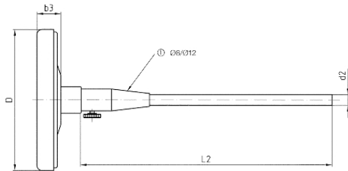
Anschluss axial
