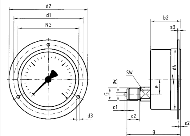
Masse (mm)
