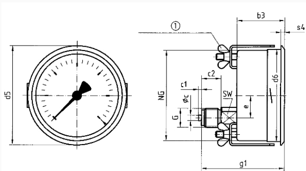
Anschluss axial, exzentrisch, 3-Kantfrontring mit Bügelbefestigung
