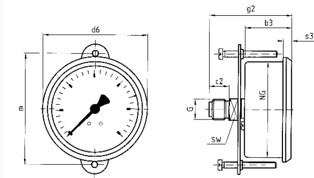
NG 40/50/63 – Anschluss axial, 3-Kantfrontring mit Bügelbefestigung
