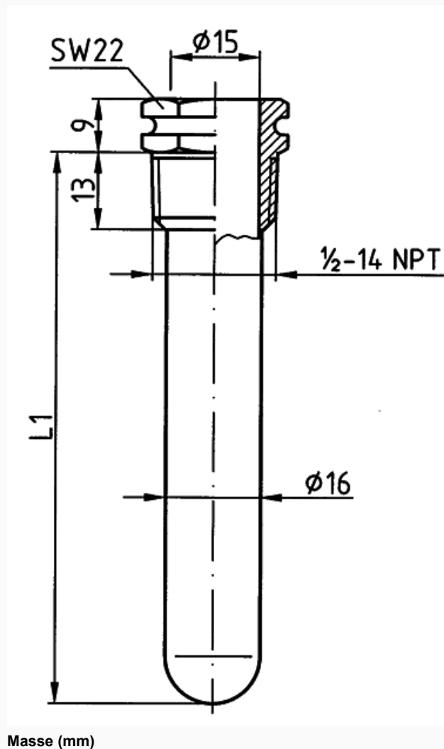
Tauchhülse ½" 15 x 16 mm
