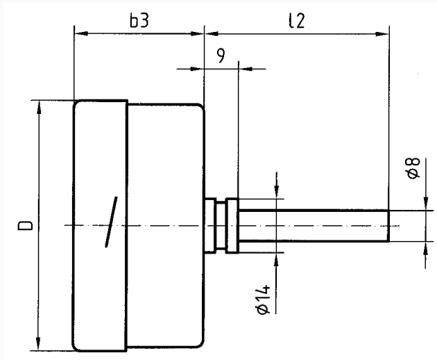
Maße (mm)
