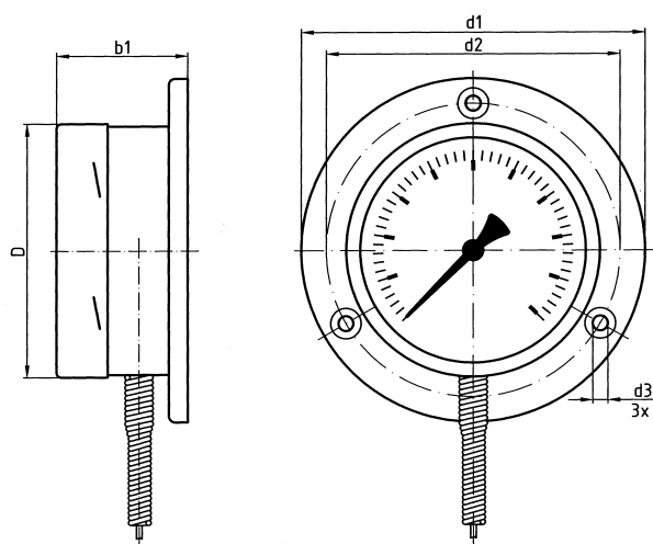
Maße (mm)
