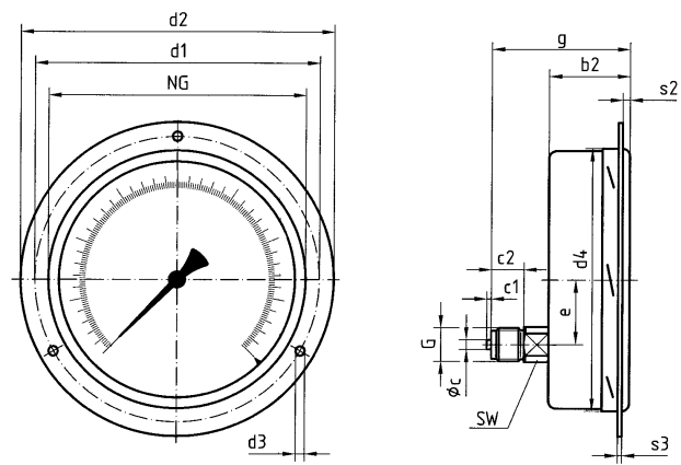
NG 160 – Anschluss axial exzentrisch, 3-Lochfrontflansch
