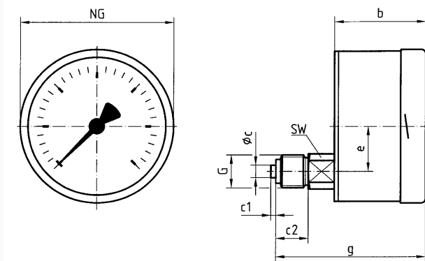
Maße (mm)
