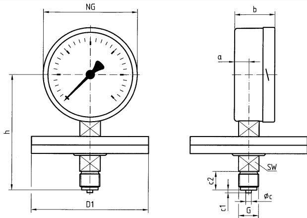
Anschluss radial, Messflansch \varnothing 160
