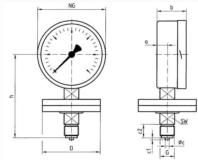
Maße (mm)
