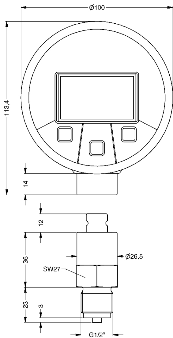
Digitalmanometer DIM 30
